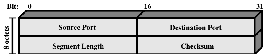
(b) UDP Header
