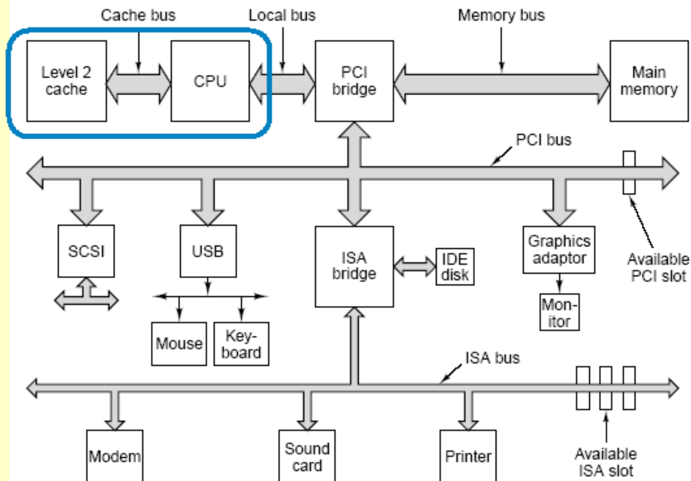
Fig. 3-50 [Tane99]
