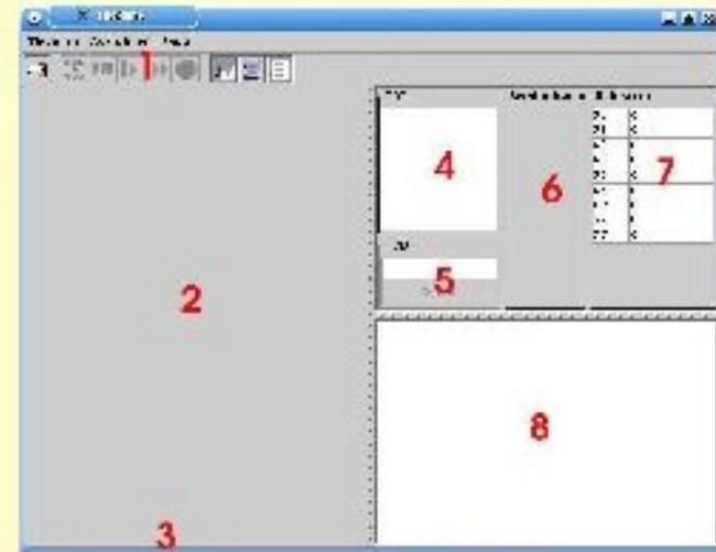
Titokoneen käyttöliittymä
