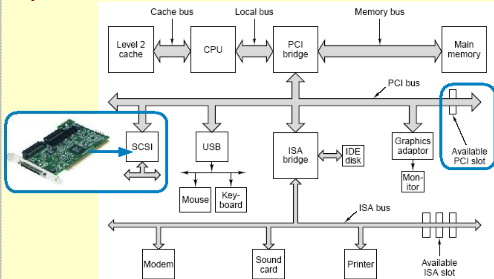
Fig. 3-50 [Tane99]
