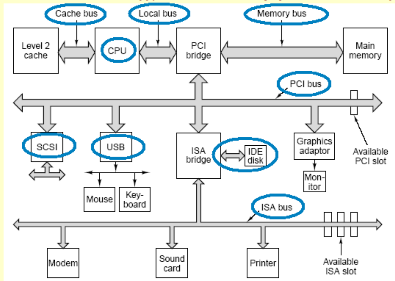
Fig. 3-50 [Tane99]
